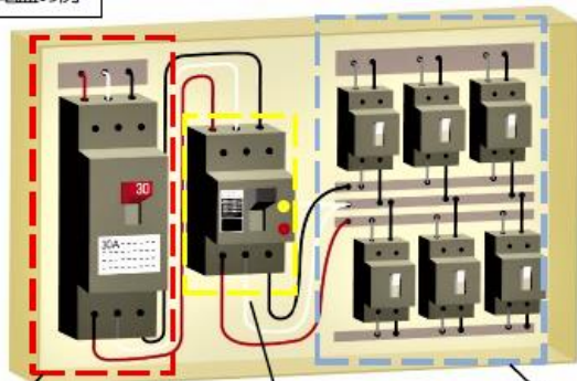
单相3線式分電盤の例
